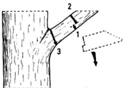
Figura 14 - Detalhe dos cortes para orientação da queda. (Michau,1998)
